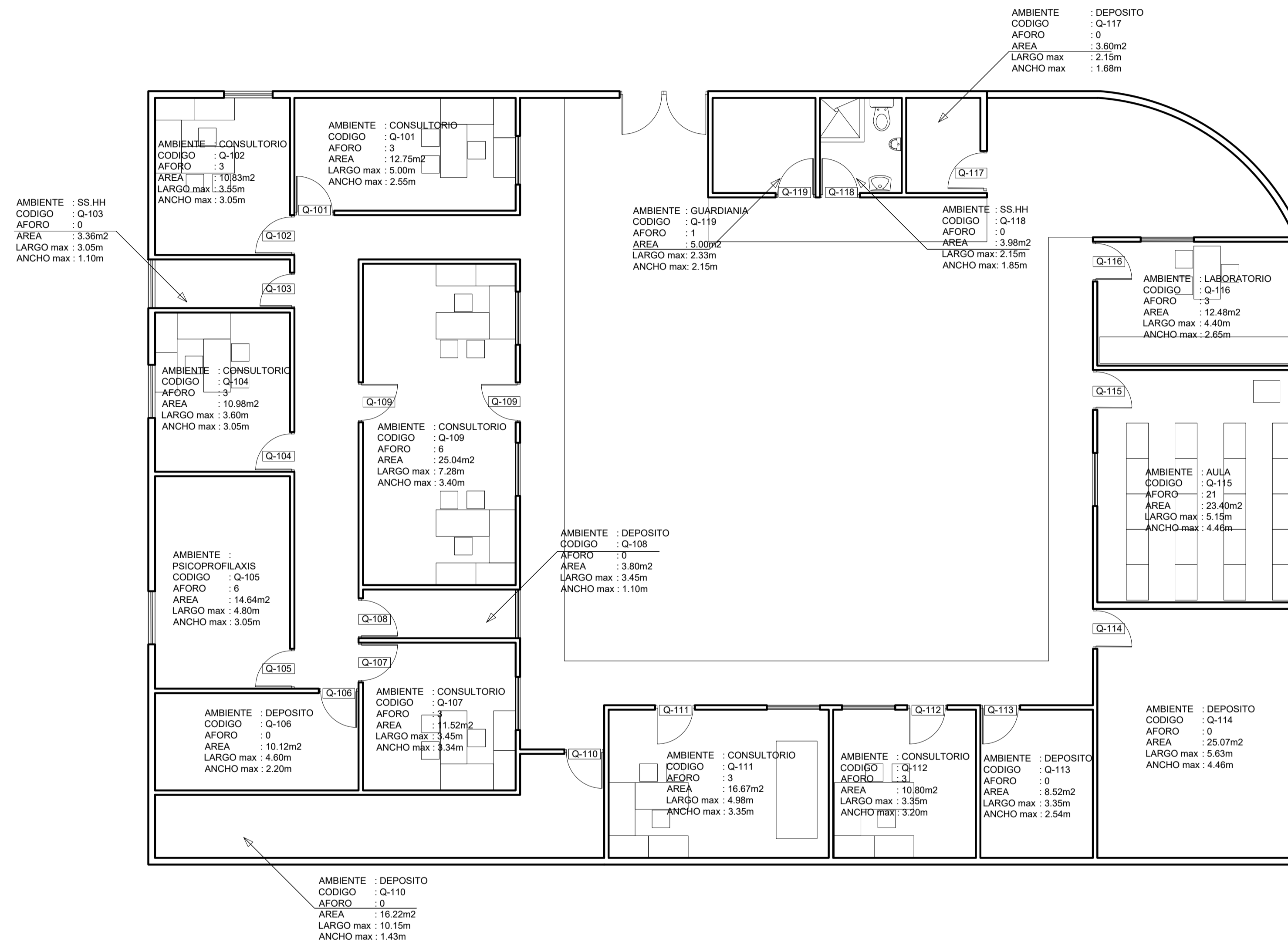
PRIMERA PLANTA AREA TECHADA = 316.92m 2 AFORO = 55 ESCALA 1:100
